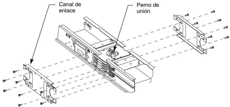
Figura 4: Instalación de los canales de enlace
