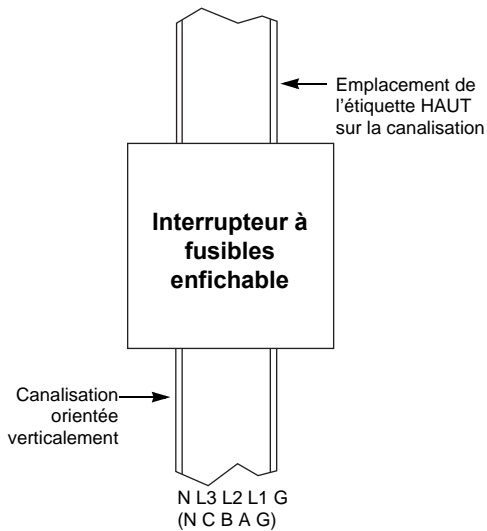
Figure 5 : Schéma de l'interrupteur à fusibles enfichable
