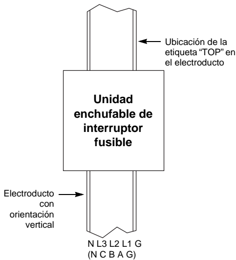
Figura 5: Diagrama de la unidad enchufable de interruptor fusible
