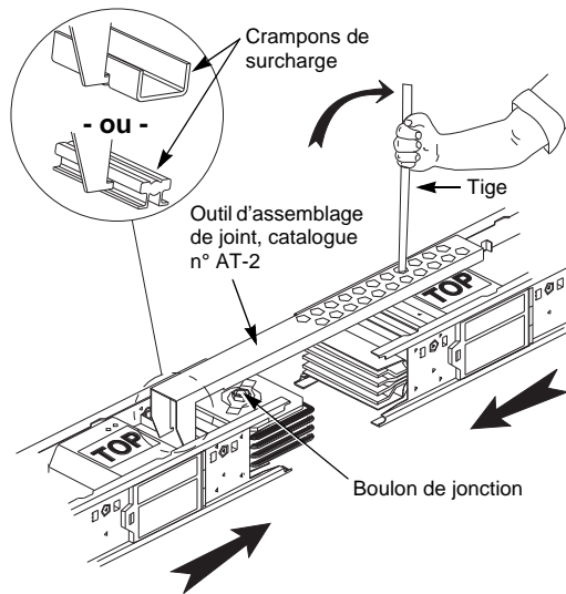
Figure 2 : Assemblage de jonctions
