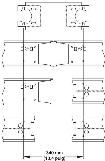
Figura 3: Separación para configuraciones varias de los extremos de unión
