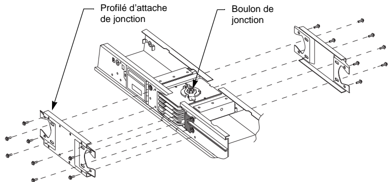
Figure 4 : Installation des profilés d'attaches de jonction
