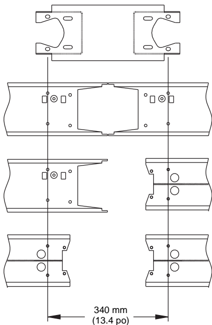
Figure 3 : Espacement des diverses configurations d'extrémités de jonction
