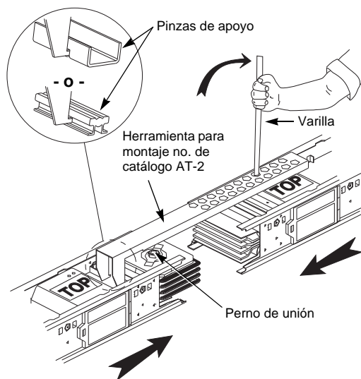
Figura 2: Ensamble de unión
