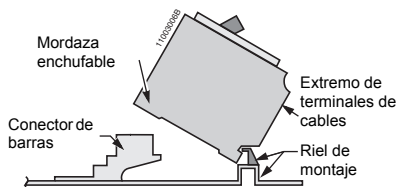
Fig 6: Interruptor automático Homeline estándar
