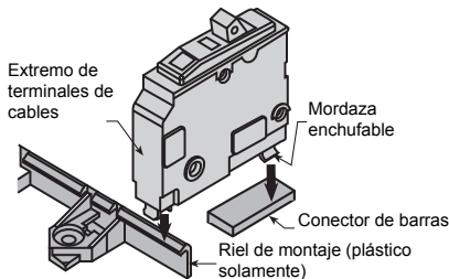
Fig 4: Interruptor automático QO estándar
