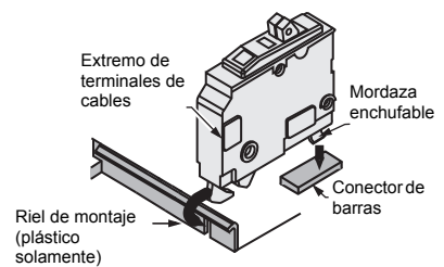
Fig 5: Interruptor automático QO en tándem
