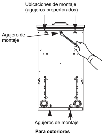
Fig 2: Montaje para sobreponer
