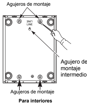
Fig 3: Montaje para empotrar
