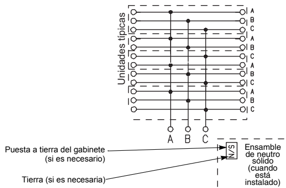
Figura 7: Alambrado típico—Zapatillas principales (400 A a )
