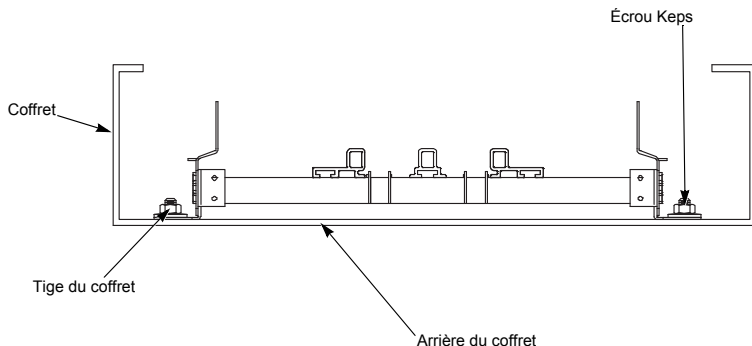
Figure 1 : Montage de l'intérieur dans des coffrets de la marque Square D
