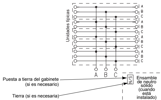
Figura 6: Alambrado típico—Zapatillas principales (225 A, 600 A, 800 A y 1 200 A)
