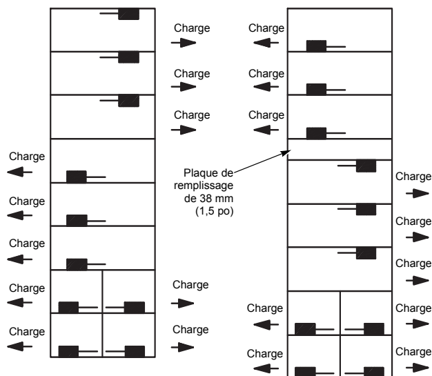
Figure 4 : Positionnement des unités à simple et double manette (haut ou bas)
