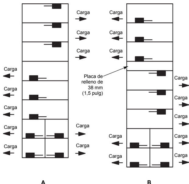
Figura 4: Posicionamiento de las unidades de una y dos palancas recomendado
