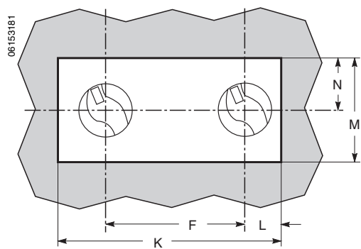
Front-panel Cutout
