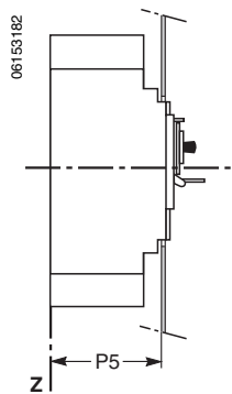
Dimensions
