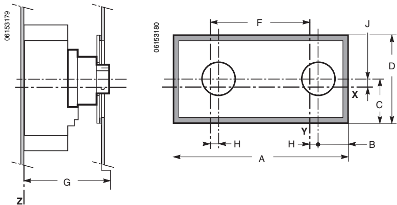
Dimensions
