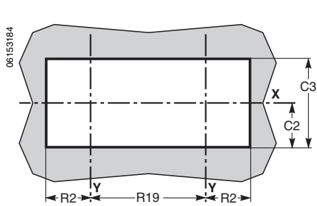
Front-panel Cutout
