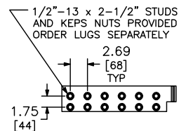
LUG LANDING PAD DETAIL
