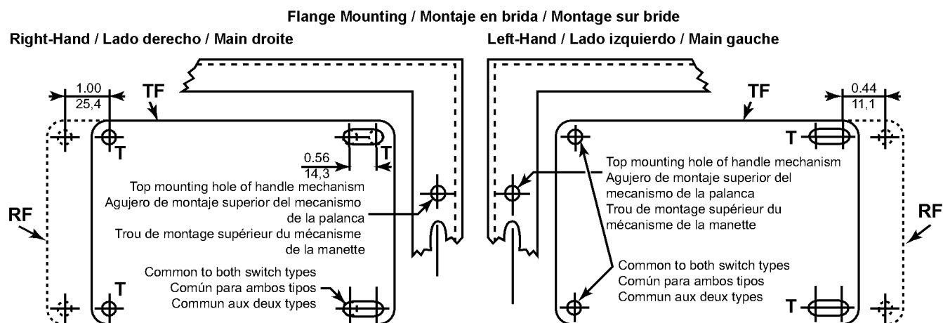
Figure / Figura / Figure 7 : Replacing Type RF with Type TF / Sustitución de un desconectador tipo RF con uno tipo TF / Remplacement d'un type RF par un type TF
