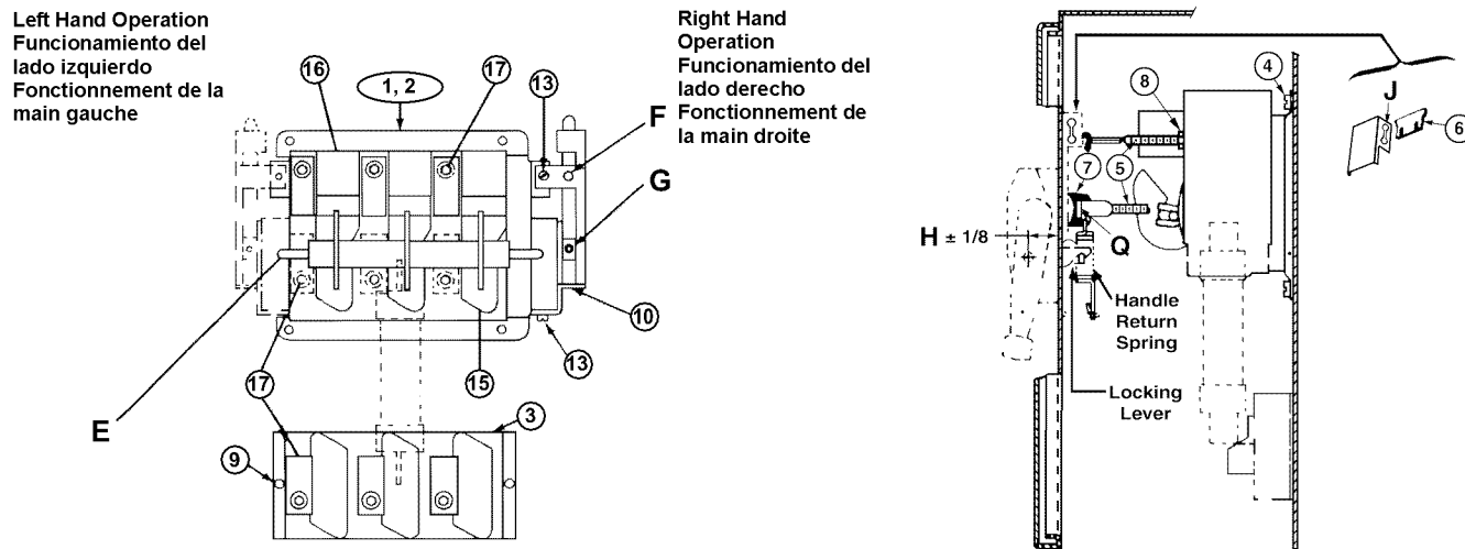
Figure / Figura / Figure 5 : Type TF3 Disconnect Switch / Desconectador seccionador tipo TF3 / Sectionneur type TF3
