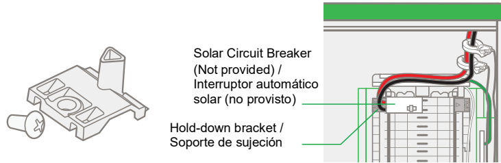
Figure / Figura 26: Connection of the Inverter to the Energy Center / Conexión del inversor al Centro de Energía
