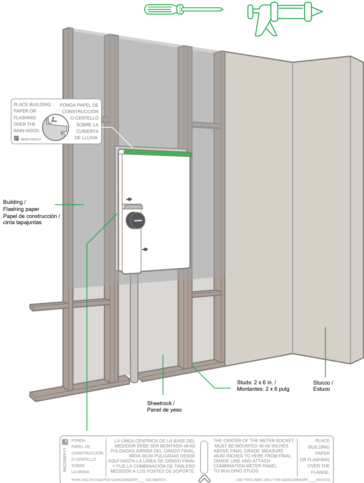
Figure / Figura 23: Energy Center Complete Installation View / Vista de la instalación completa del Centro de Energía
