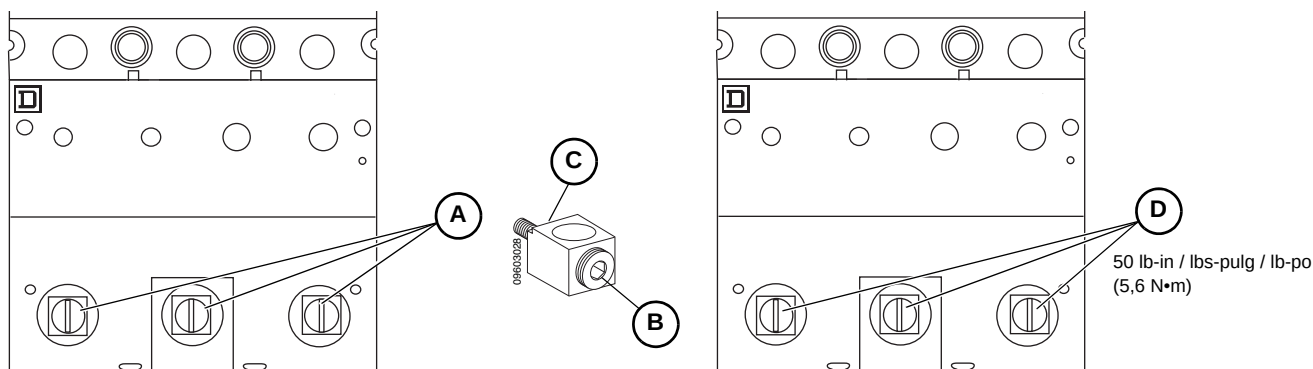
FIG. 10 : Wiring Installation / Instalación de los cables / Raccordement du câblage
