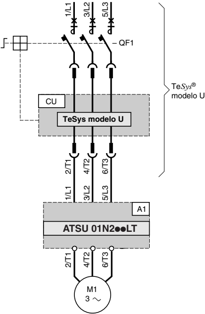
Cableado de potencia
