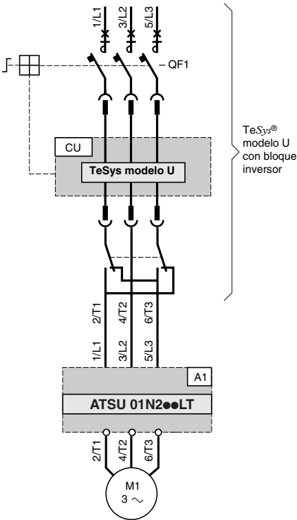
Cableado de potencia con bloque inversor
