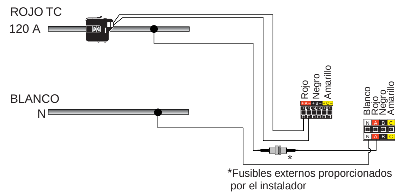
Figure 8: Instalación con 1 fase y 2 hilos
