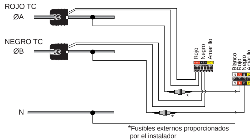
Figure 7: Instalación con 1 fase y 3 hilos
