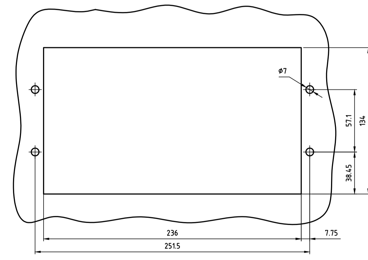
Tafelausschnitt Dècoupe du panneau Panel cut-out M 1:2
