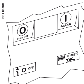
Schalter AUS, Speicher gespannt, nicht „einschaltbereit“
