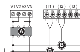
1PH3W multi L-N 2LVCS
