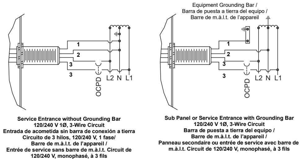
FIG. 6 : Typical AC Surge Module Wiring Connection Diagrams / Diagramas típicos de conexión del alambrado del módulo de ~ contra sobretensiones transitorias / Schémas typiques de raccordement du module ca d'un SPD
