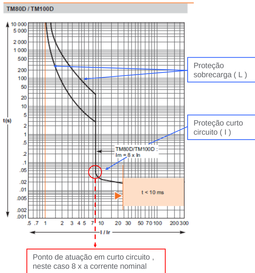
Curva de funcionamento para disparador tipo distribuição
