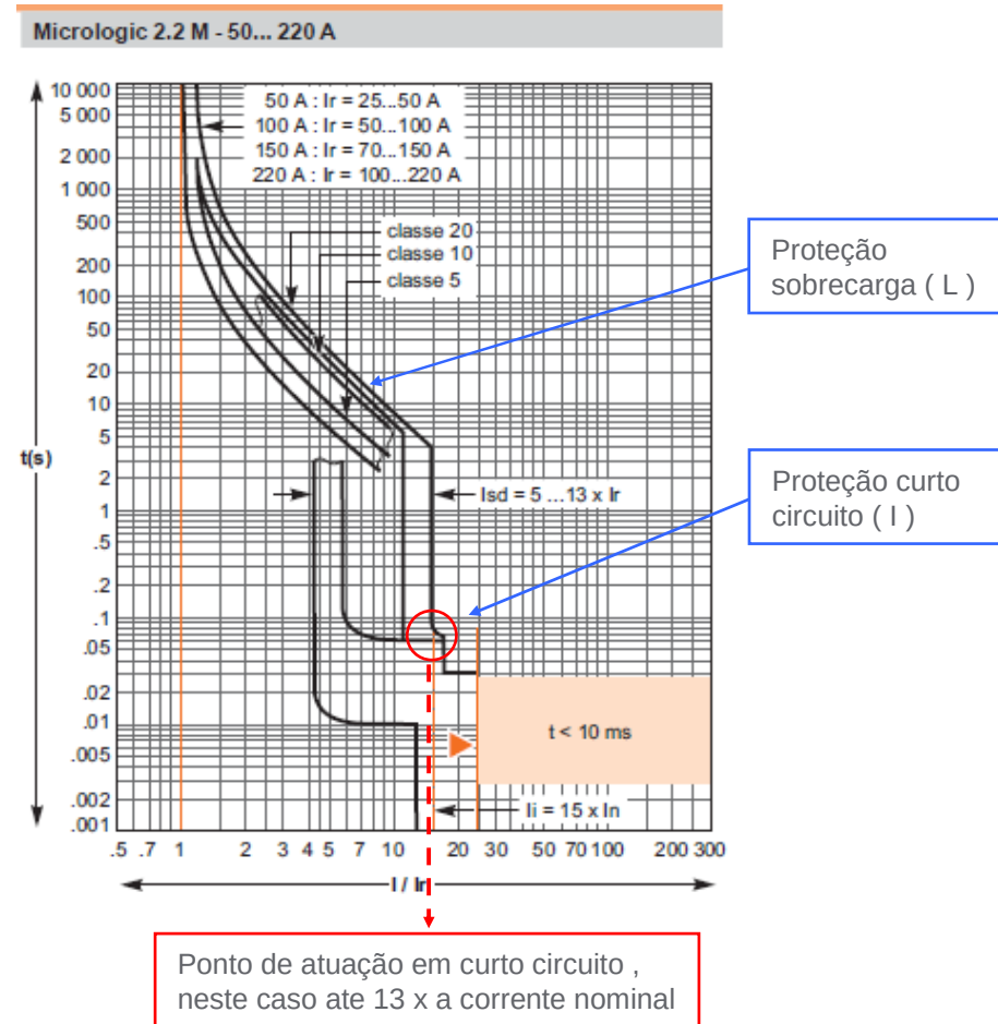
Curva de funcionamento para disparador tipo motor
