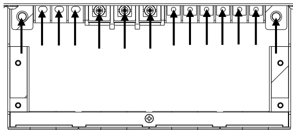
Eingangsverdrahtung 3:3 duale Zuleitung
