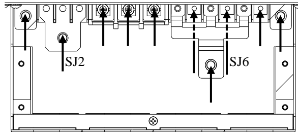
Eingangsverdrahtung 3:1 duale Zuleitung
