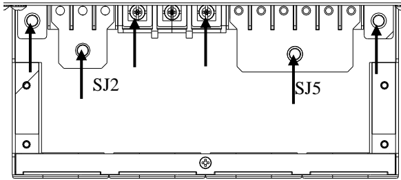
Eingangsverdrahtung 3:1 einzelne Zuleitung
