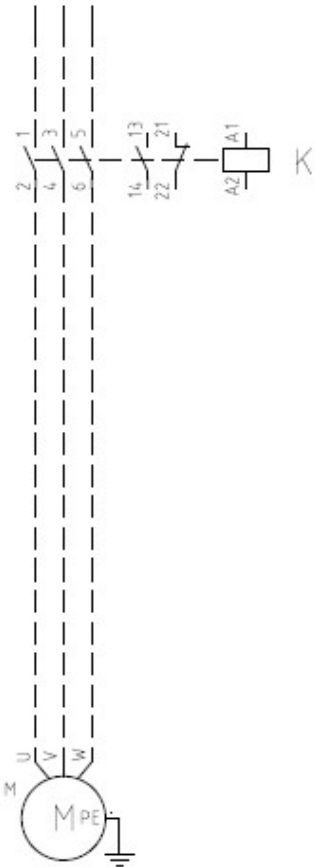
Kontaktor
