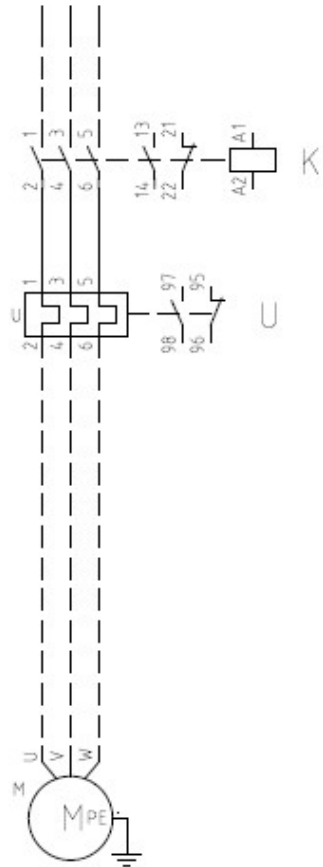
Kontaktor- motorskydd
