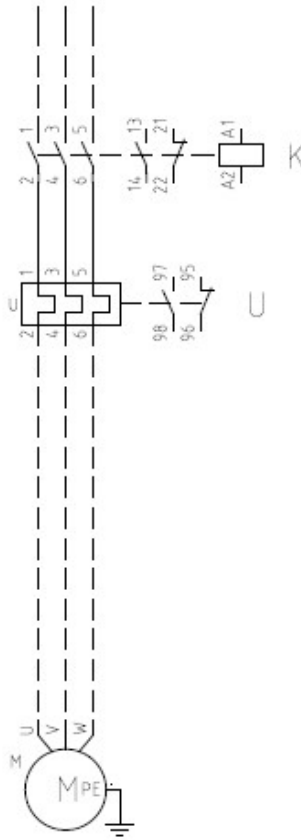
Kontaktor- motorskydd
