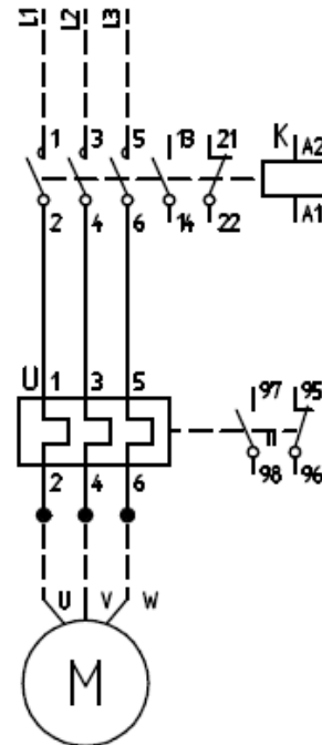
Kontakformotorskydd
