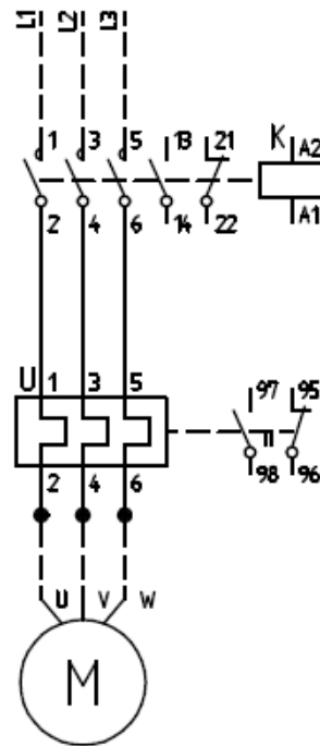
Kontakformotorskydd
