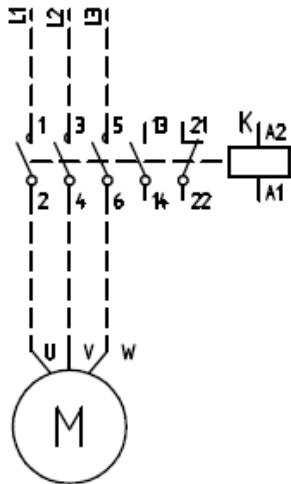
Kontaktor
