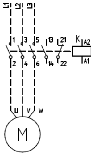
Kontaktor
